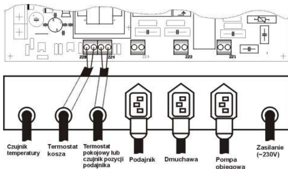
Rys. 2. Podłączenie współpracujących urządzeń.
